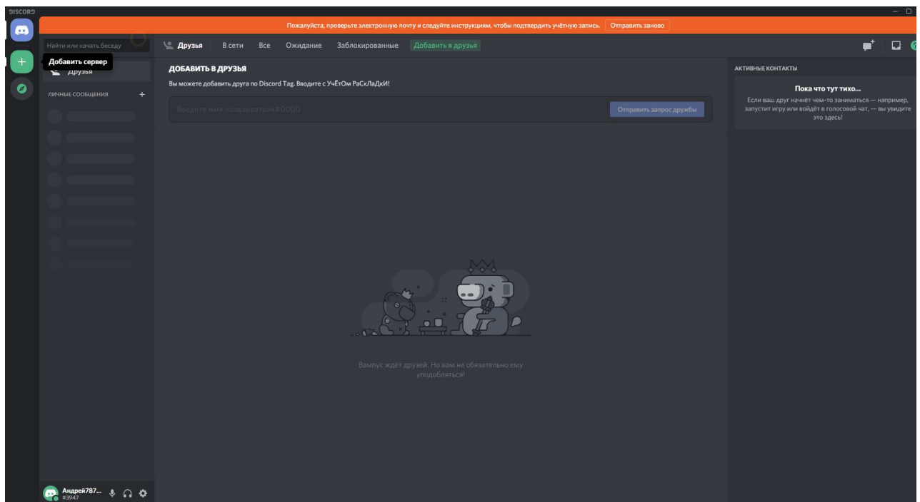
Рисунок 4 – добавление сервера
