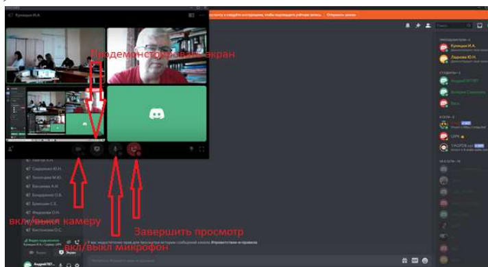
Рисунок 7 - интерфейс программы
