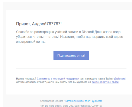
Рисунок 3 – Подтверждение почты
