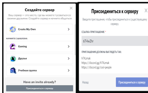
Рисунок 5- приглашение
